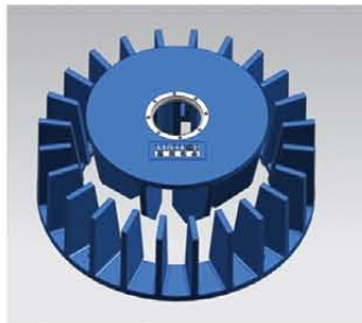
浮选机定子、转子 Flotation machine stator, rotor
